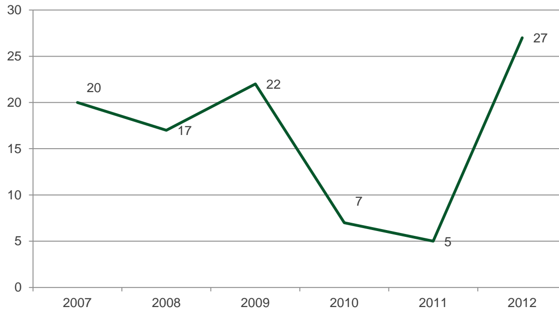
Antal overtrædelser
